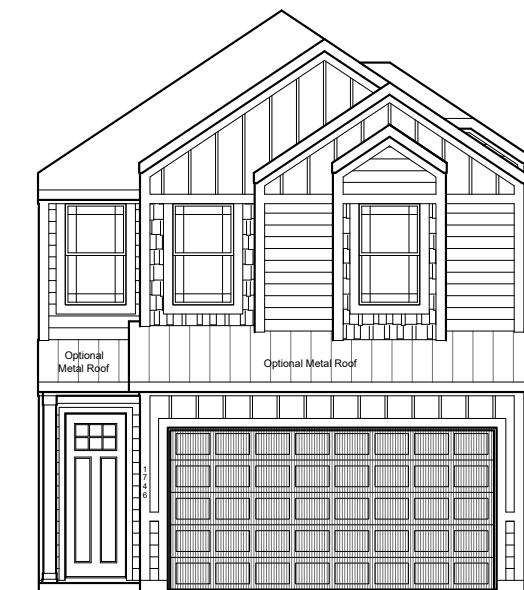
Elevation B
