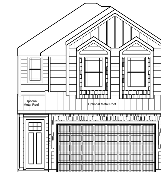
Elevation B
