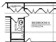
OPTIONAL BED 6 BATH 4
