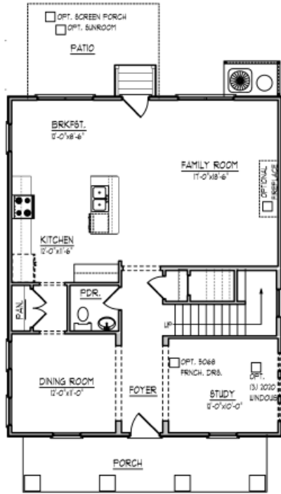
ELEVATION A
