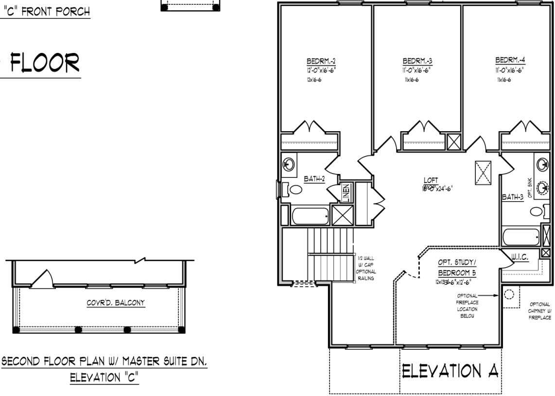
ELEVATION A
