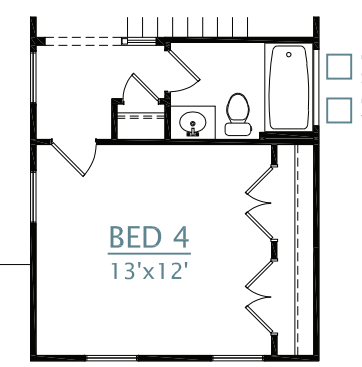
OPTIONAL BEDROOM 4
