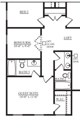
OPTIONAL GUEST SUITE
