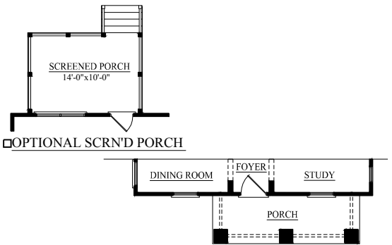
□ OPTIONAL SCRND PORCH
