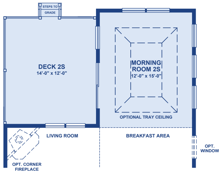
Optional Deck 2S
